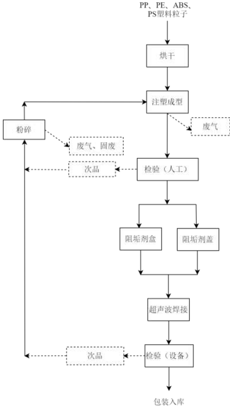
图 2-2 厨卫、电器配套产品的生产工艺流程及产污环节图 注：本项目为单种塑料粒子进行注塑成型，不涉及拌料、混料工序。 厨卫、电器配套产品的生产工艺流程及产排污说明：
