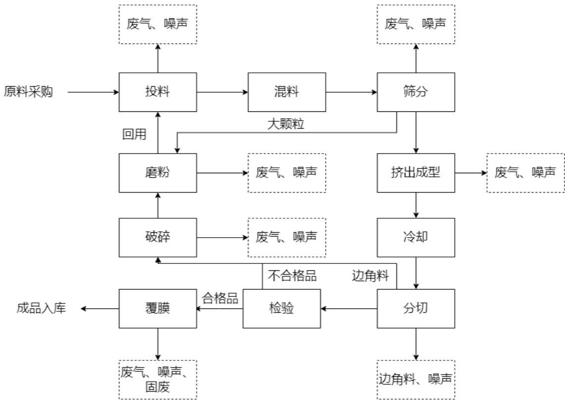
图 2-2 本项目生产工艺流程及产污环节图
