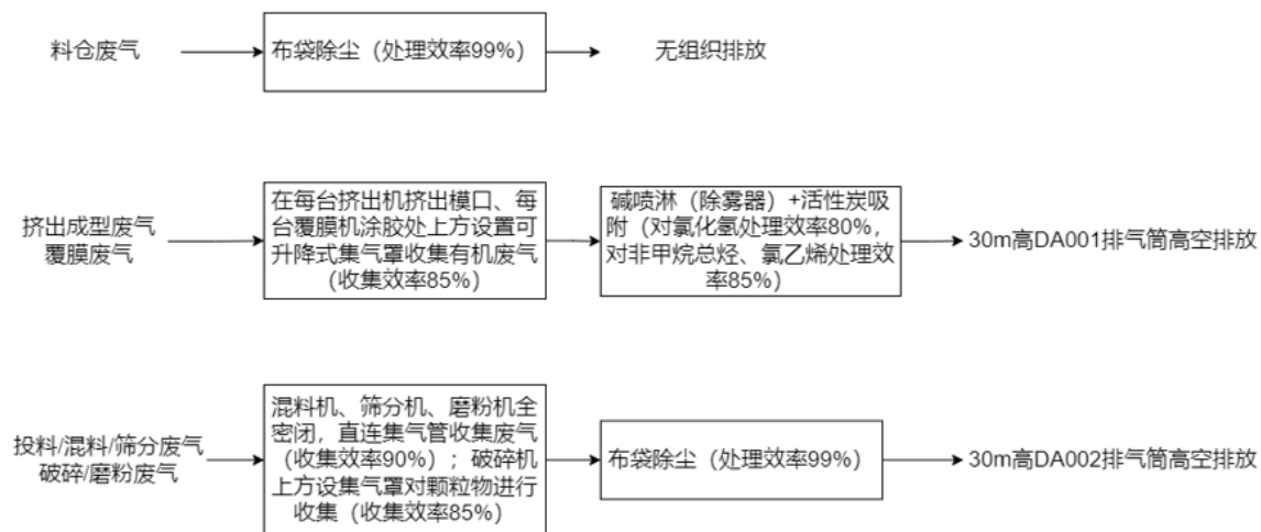
图 4-1 废气污染防治系统图
