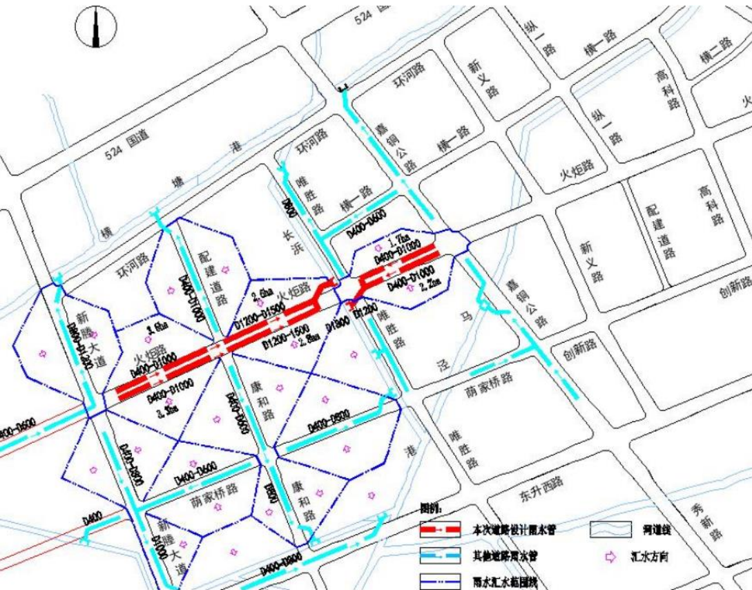
图2-6 雨水系统图
