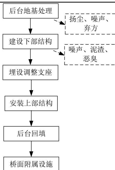
图 2-11 桥梁工程施工工艺流程图
