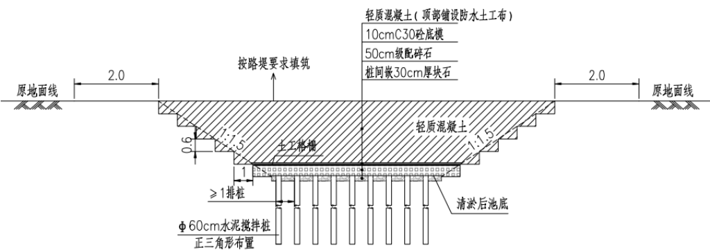
图2-5 河道填筑图
