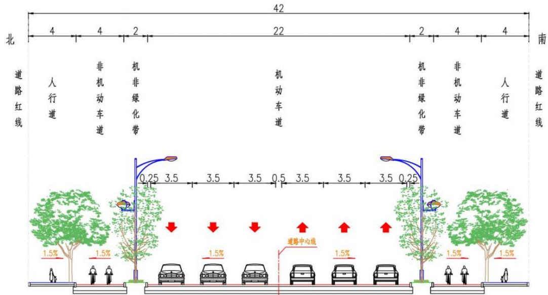
图 2-1 火炬路（新塍大道-嘉铜公路）标准横断面设计图
