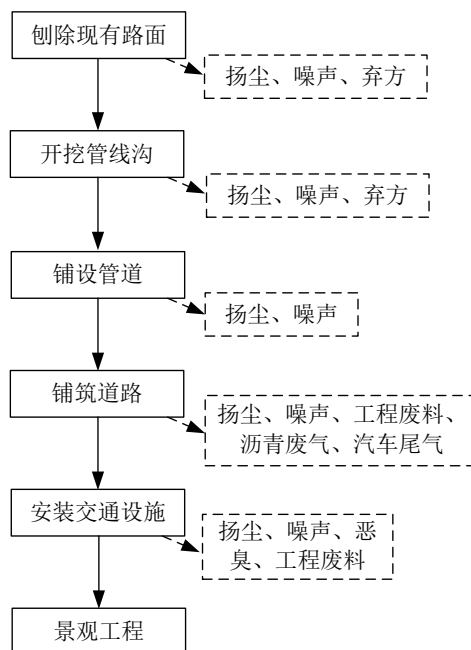
图 2-10 道路工程施工工艺流程图
