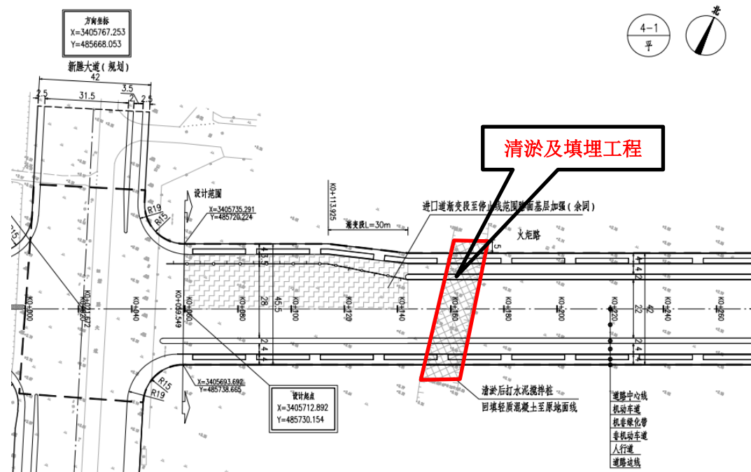
图2-4 清淤及填埋位置图
