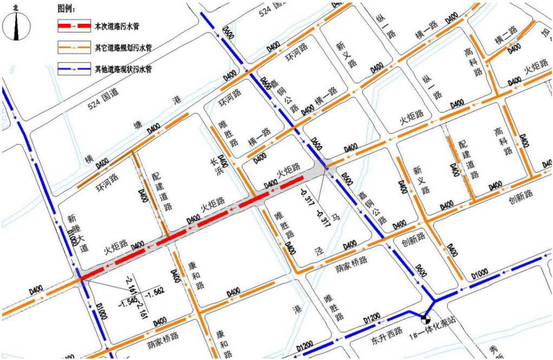
图2-7 污水系统图
