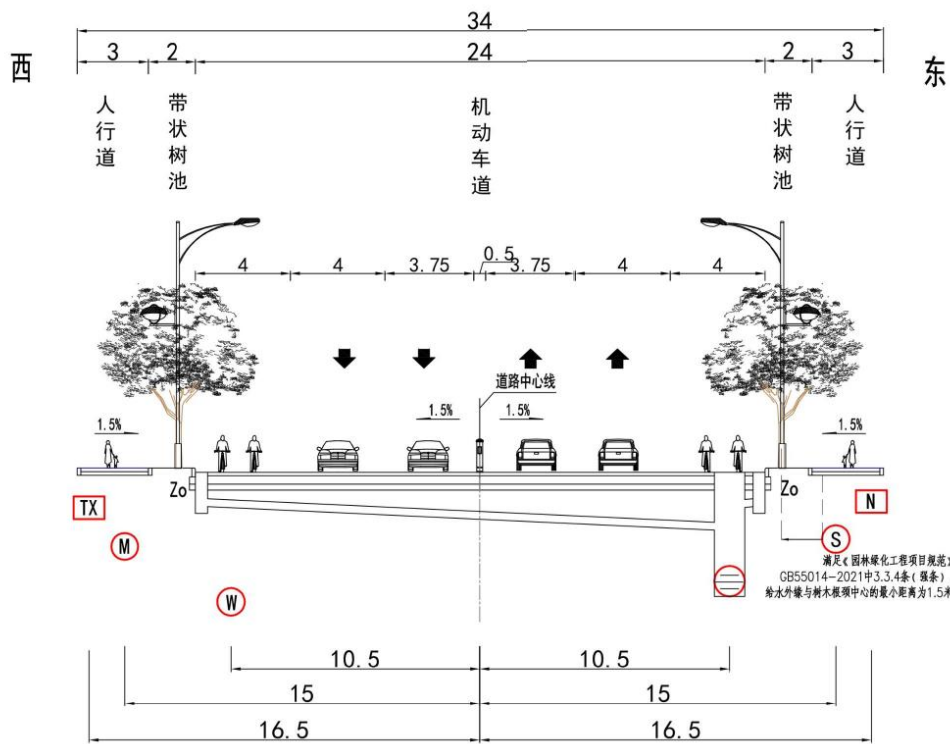
图2-9 新义路（环河路-火炬路）标准管位图
