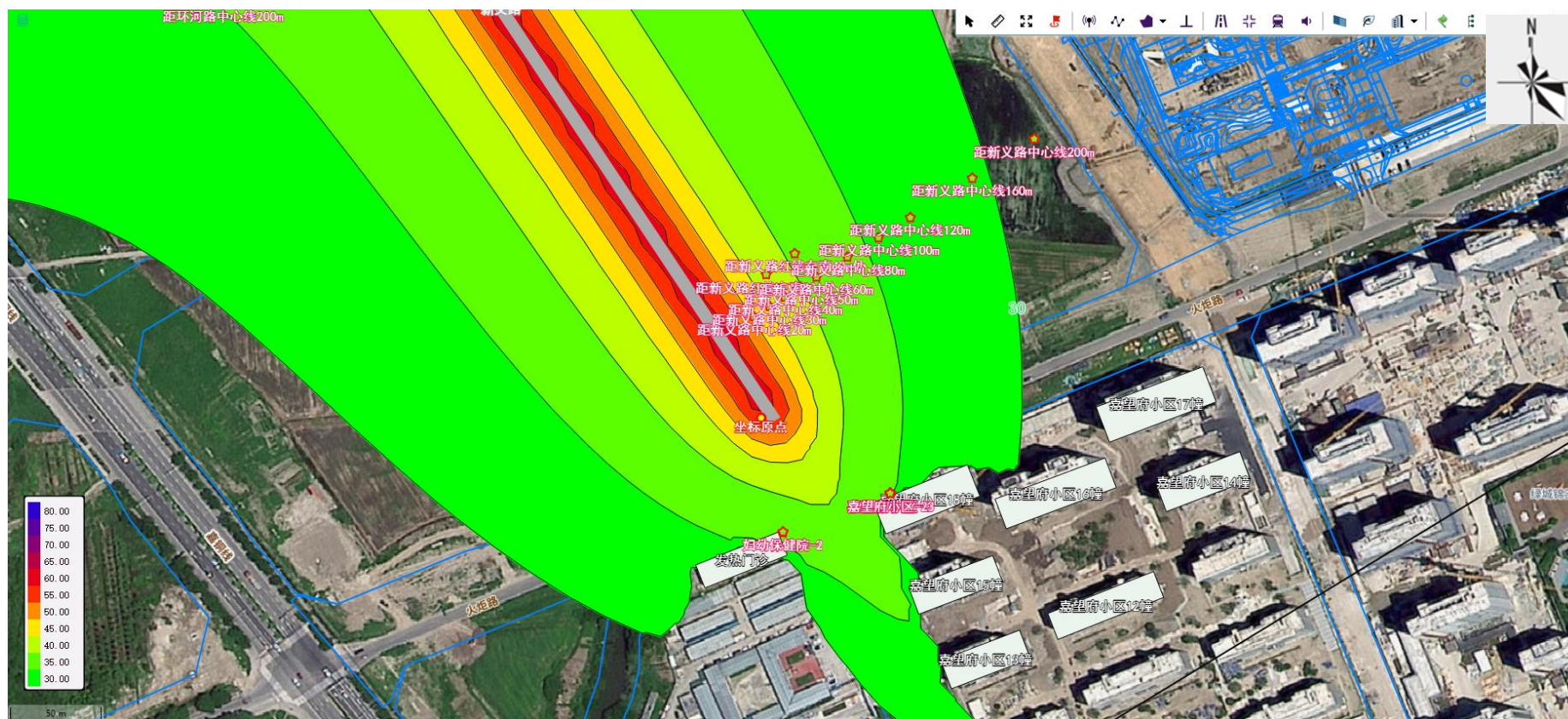
图 4-2 营运近期-夜间-水平方向噪声贡献值等声级线图（右下）
