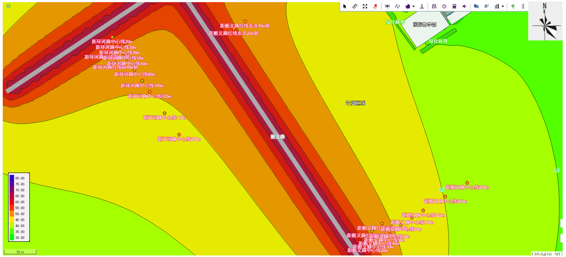
图 4-3 营运中期-昼间-水平方向噪声贡献值等声级线图（左下）
