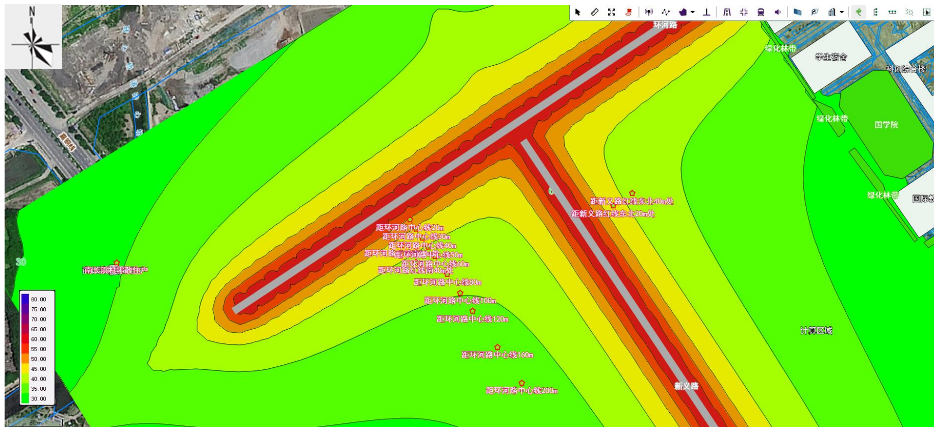
图 4-6 营运远期-夜间-水平方向噪声贡献值等声级线图（左上）
