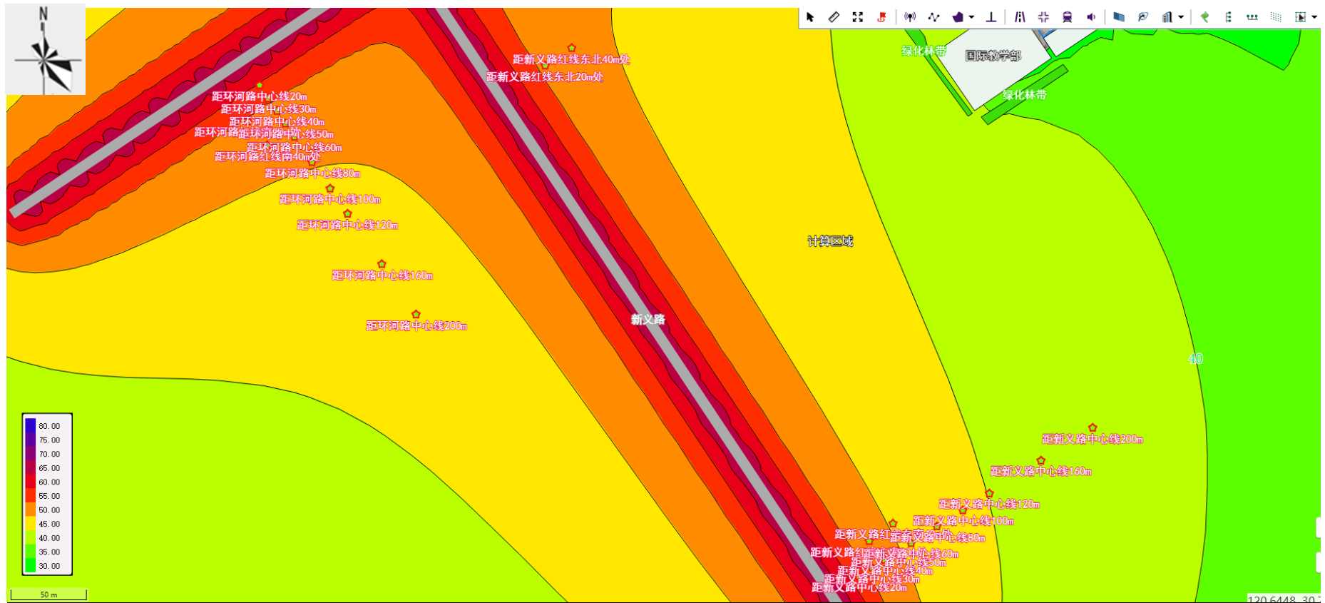
图 4-1 营运近期-昼间-水平方向噪声贡献值等声级线图（左下）
