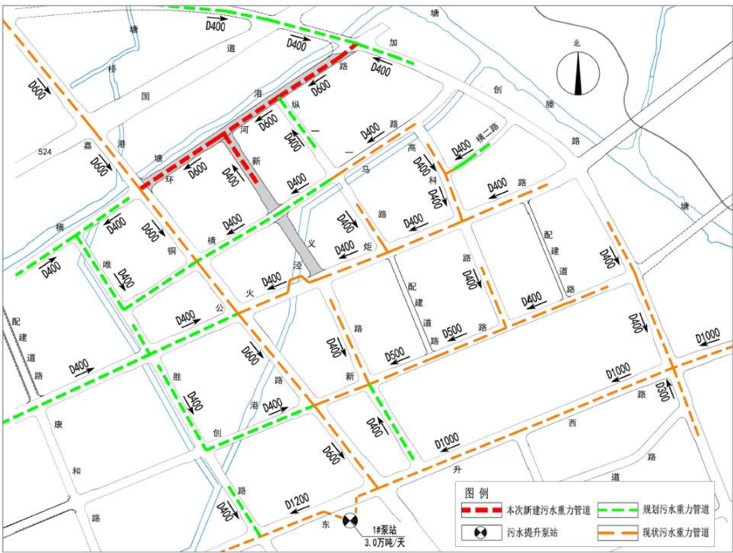
图2-7 污水主干走向示意图
