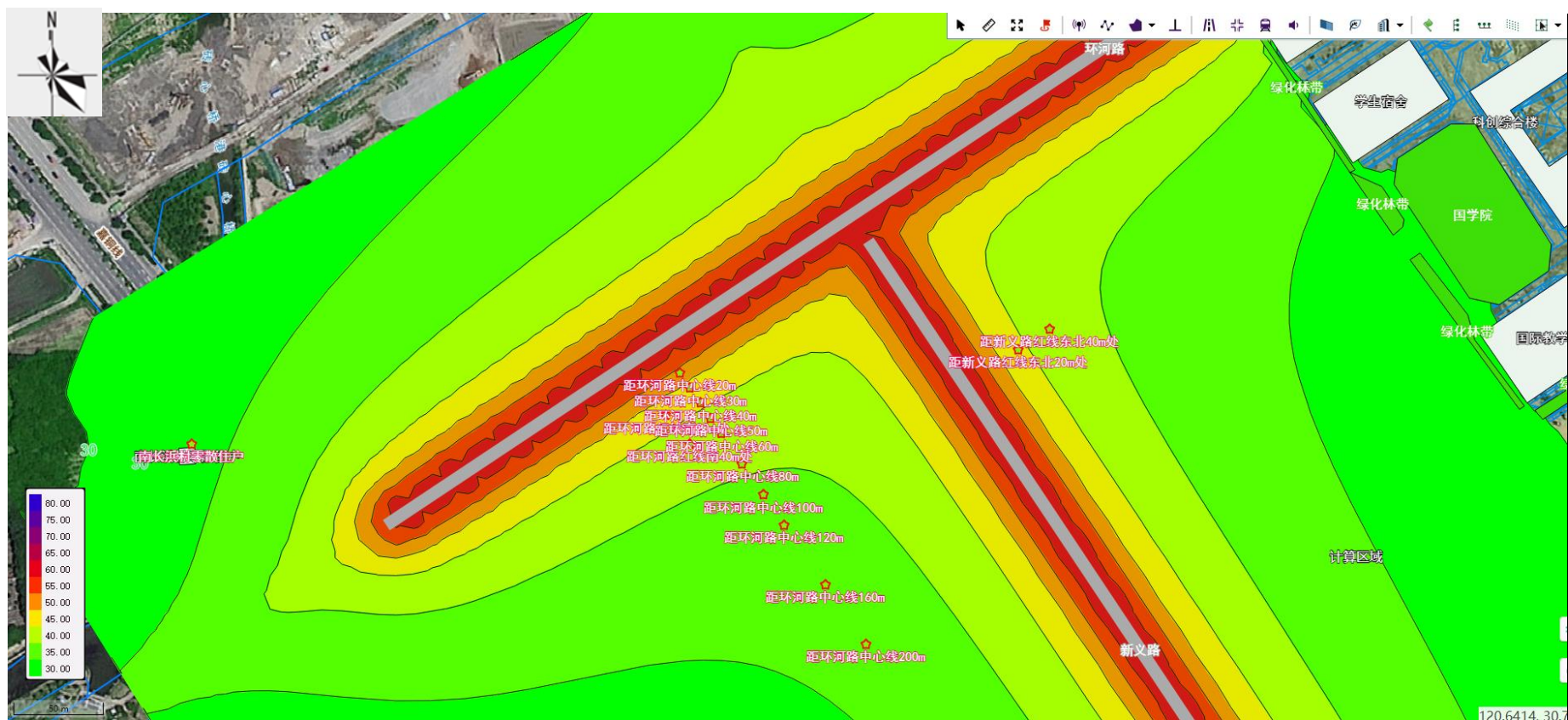
图 4-4 营运中期-夜间-水平方向噪声贡献值等声级线图（左上）
