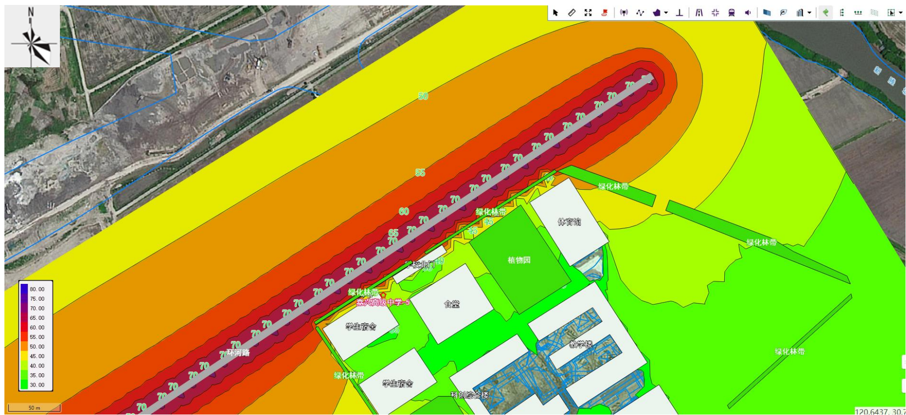
图 4-5 营运远期-昼间-水平方向噪声贡献值等声级线图（右上）
