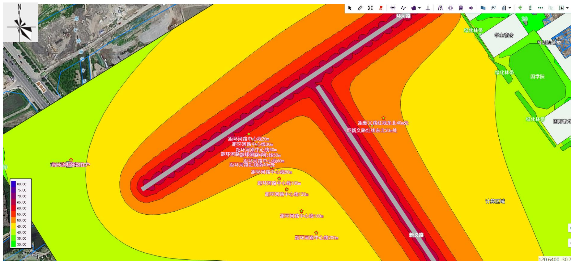
图 4-1 营运近期-昼间-水平方向噪声贡献值等声级线图（左上）
