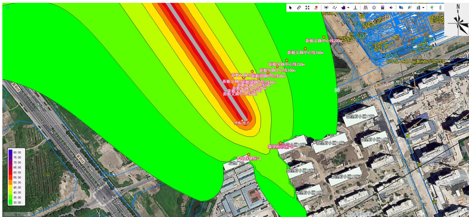
图 4-4 营运中期-夜间-水平方向噪声贡献值等声级线图（右下）
