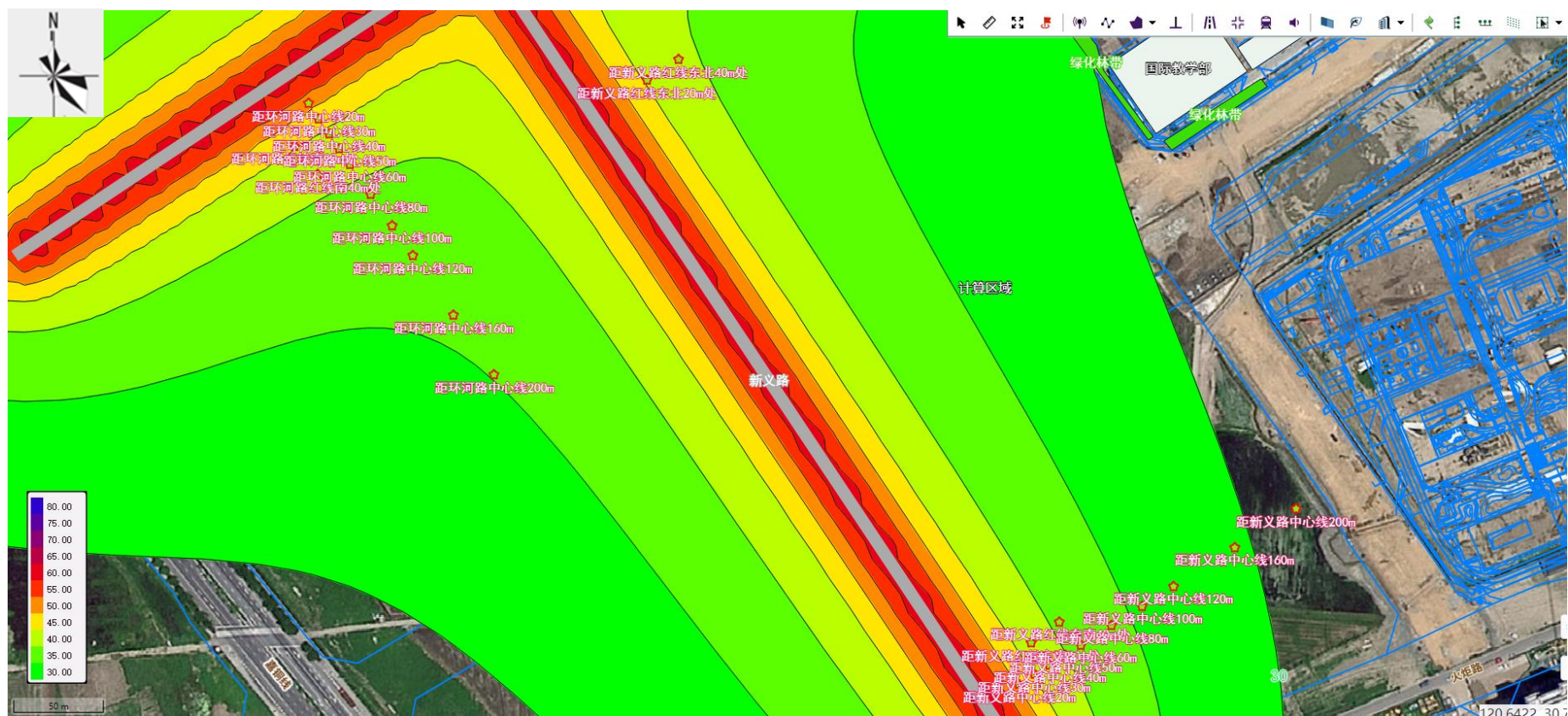
图 4-2 营运近期-夜间-水平方向噪声贡献值等声级线图（左下）
