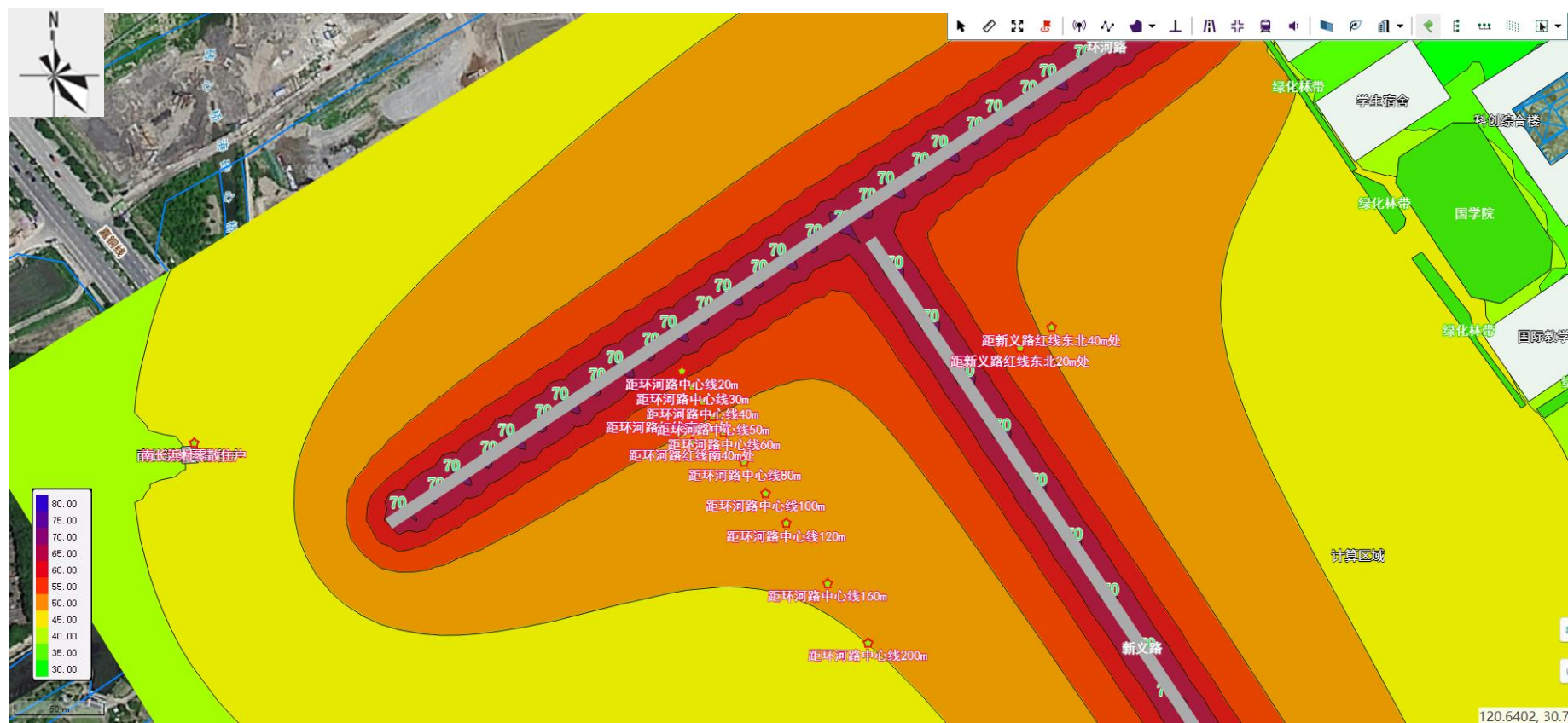
图 4-5 营运远期-昼间-水平方向噪声贡献值等声级线图（左上）
