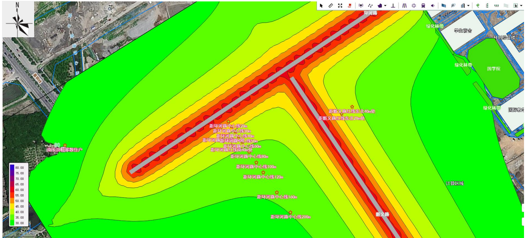
图 4-2 营运近期-夜间-水平方向噪声贡献值等声级线图（左上）
