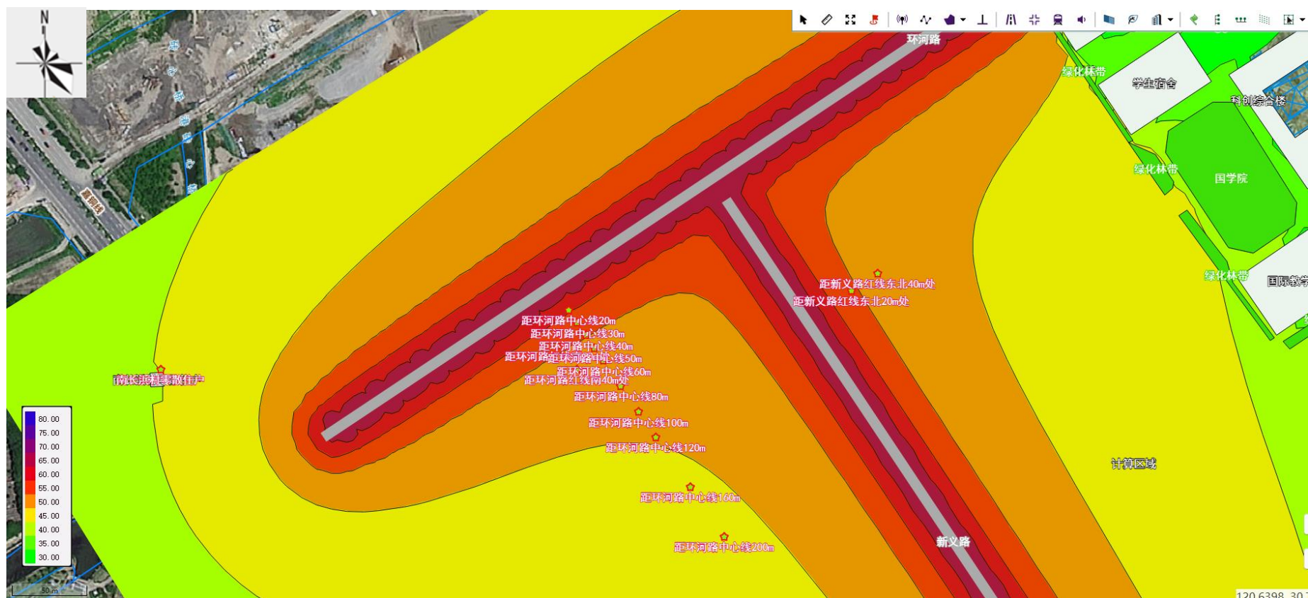
图 4-3 营运中期-昼间-水平方向噪声贡献值等声级线图（左上）
