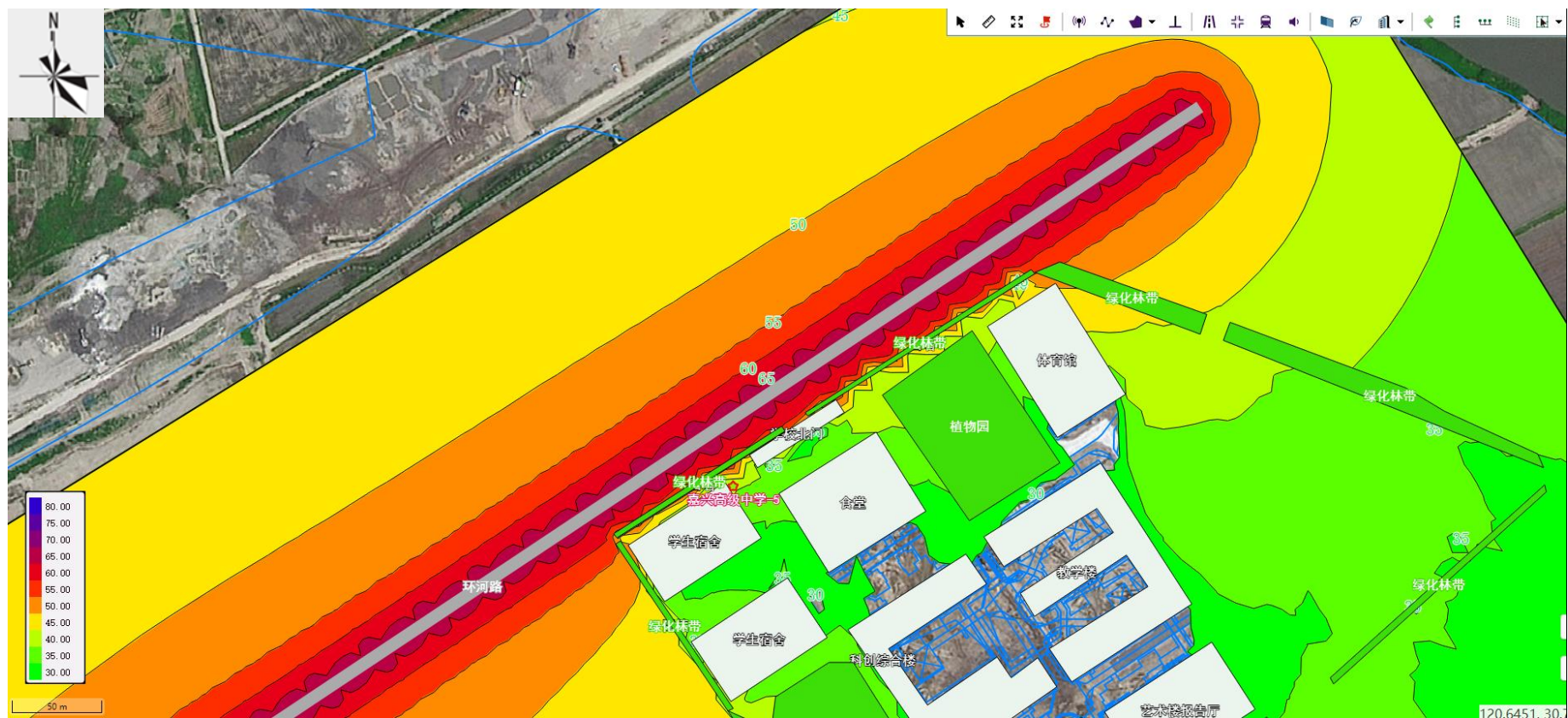
图 4-1 营运近期-昼间-水平方向噪声贡献值等声级线图（右上）
