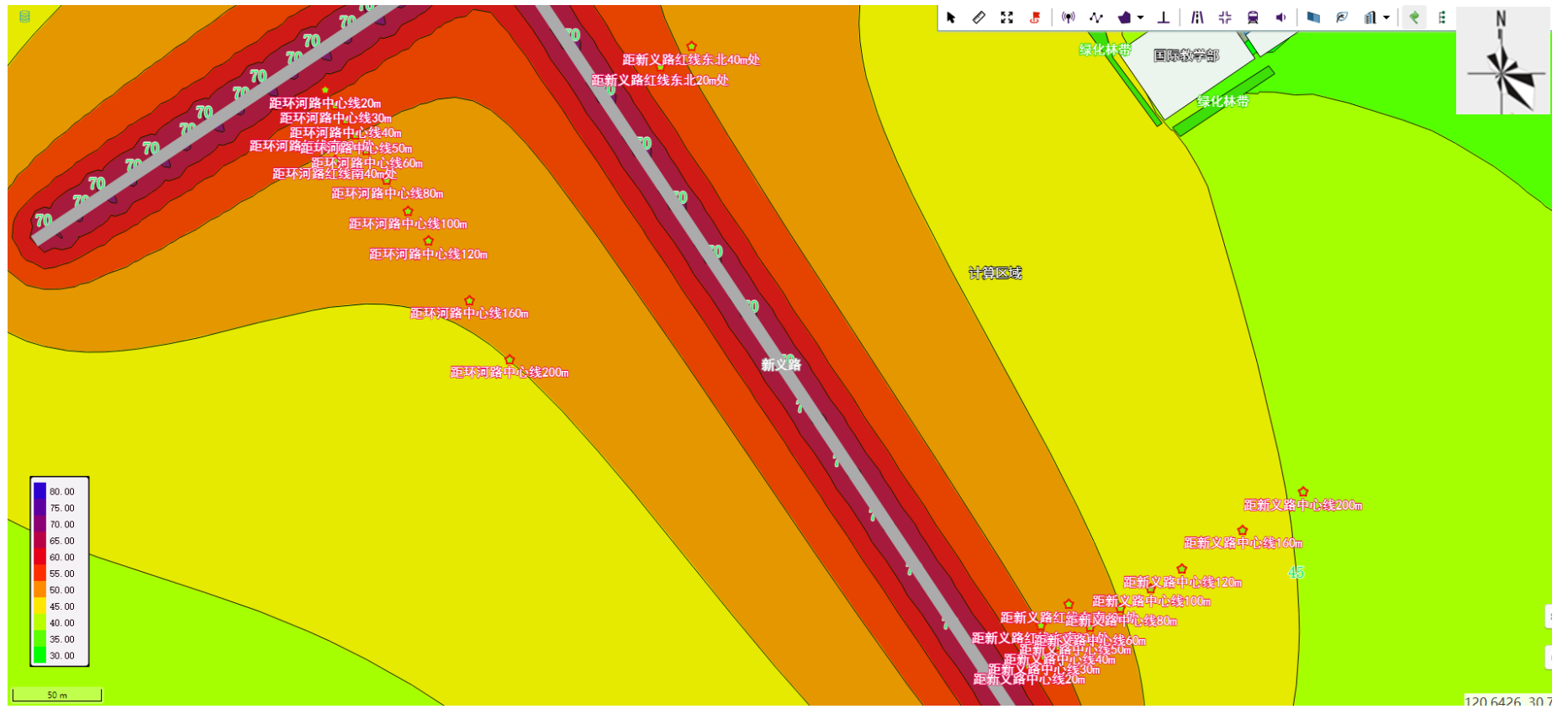
图 4-5 营运远期-昼间-水平方向噪声贡献值等声级线图（左下）
