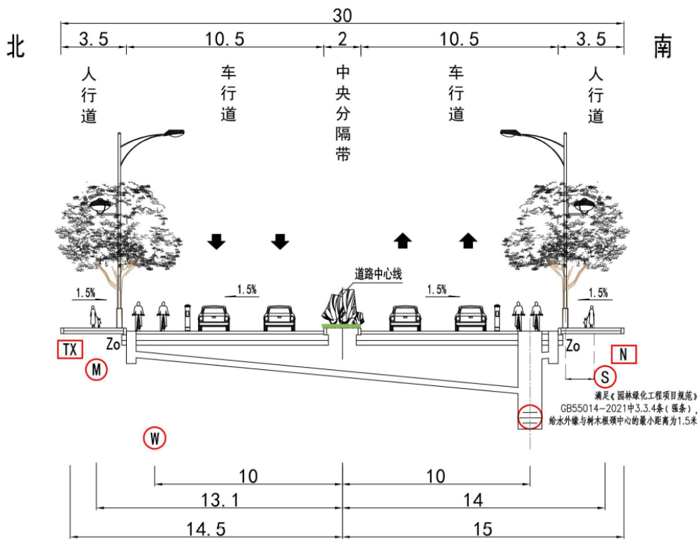
图2-8 环河路（嘉铜公路-加创路）标准管位图
