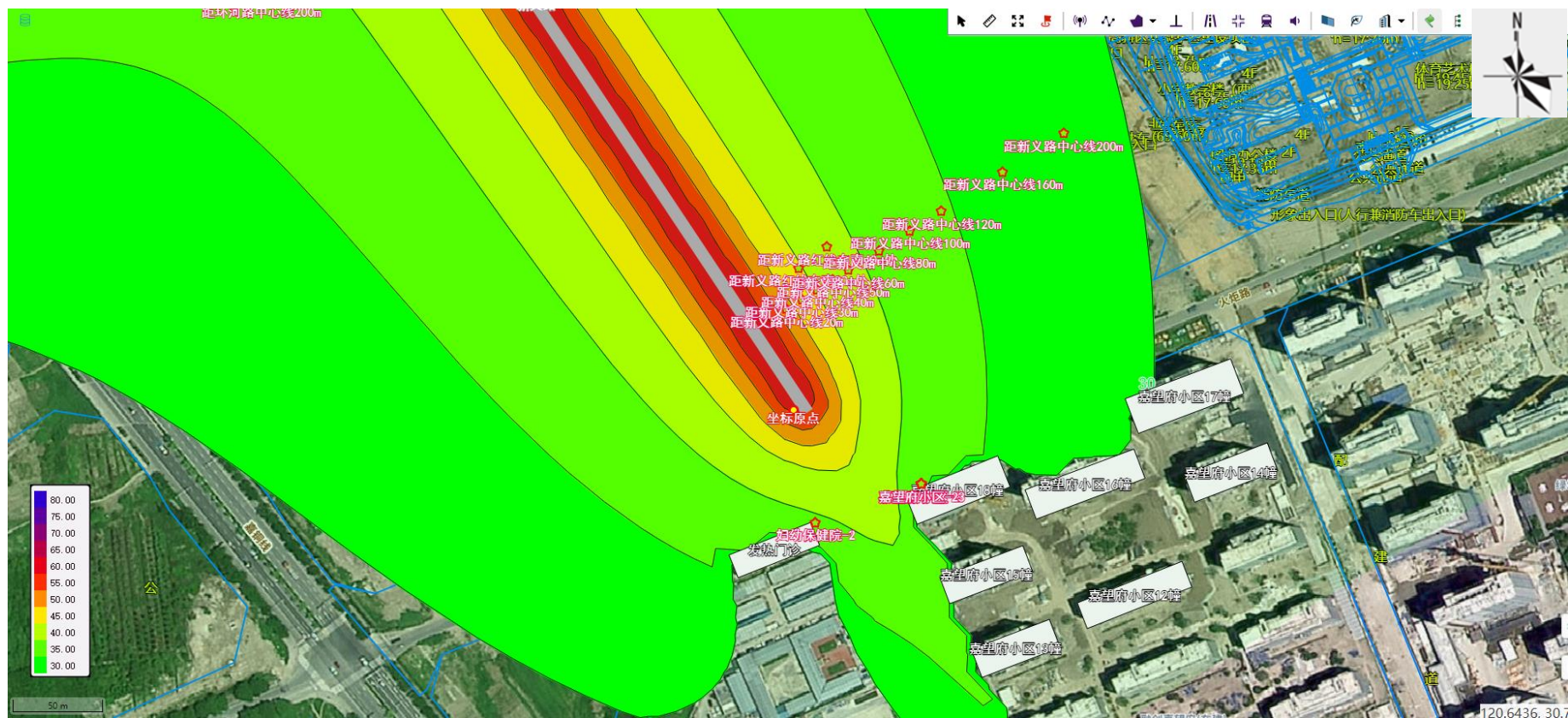
图 4-6 营运远期-夜间-水平方向噪声贡献值等声级线图（右下）
