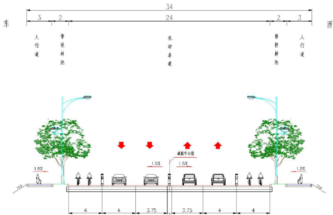
图 2-2 新义路（环河路-火炬路）标准横断面设计图
