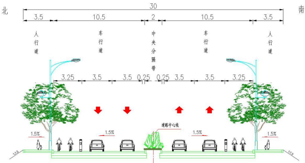
图 2-1 环河路（嘉铜公路-加创路）标准横断面设计图
