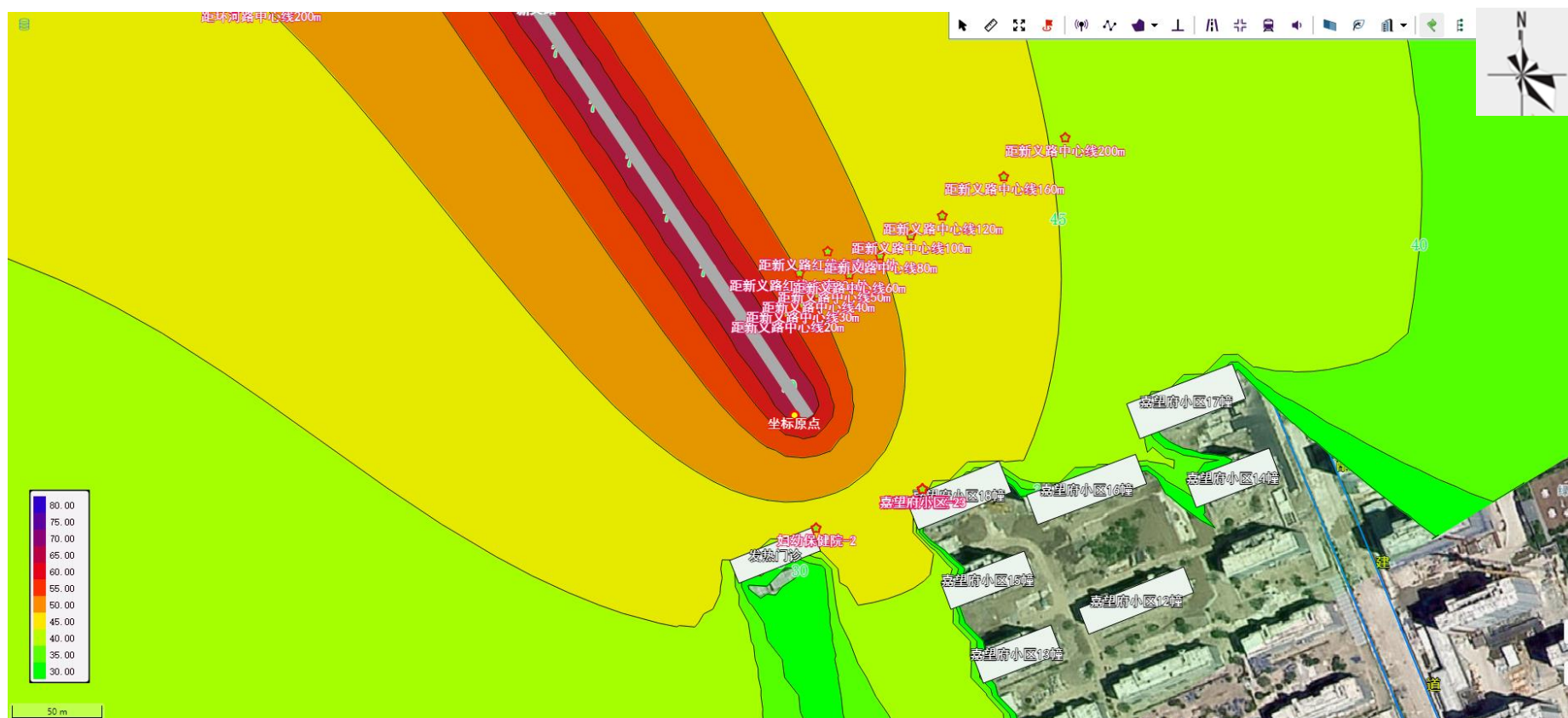
图 4-5 营运远期-昼间-水平方向噪声贡献值等声级线图（右下）
