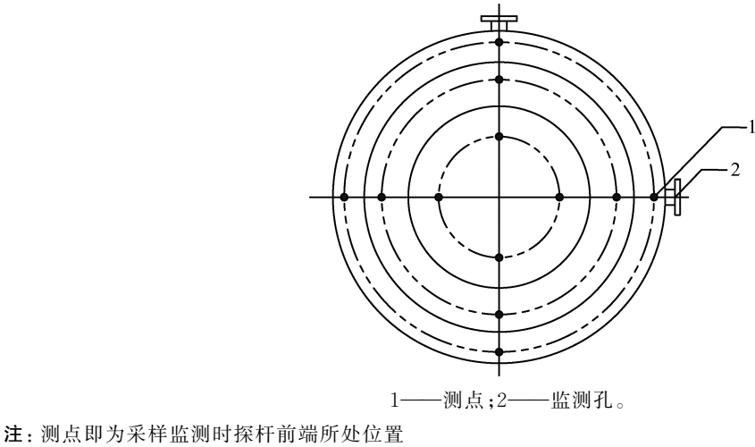
图 3 圆形断面测点与监测孔示意图
