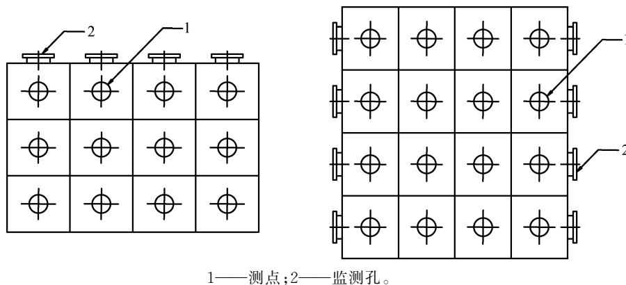
图4 矩形断面测点与监测孔示意图
